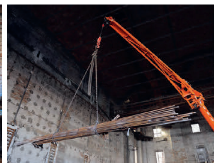
МОНТАЖ МЕТАЛЛОКОНСТРУКЦИЙ
